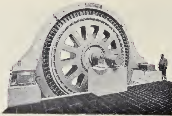
Alternatore monofase di 750 cavalli.
